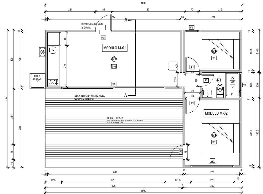
PLANTA DE ARQUITECTURA
