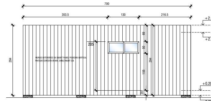
ELEVACION LATERAL DERECHA
