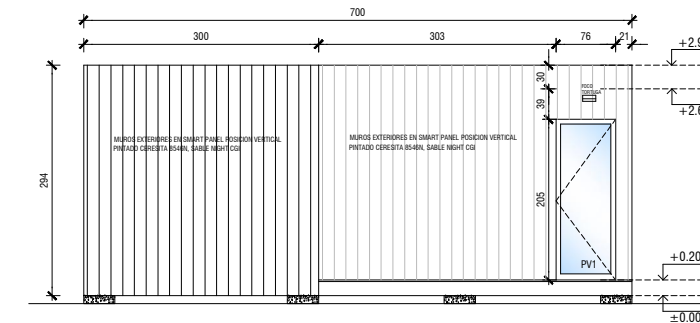
ELEVACION LATERAL IZQUIERDA
