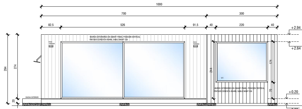
ELEVACION PRINCIPAL
