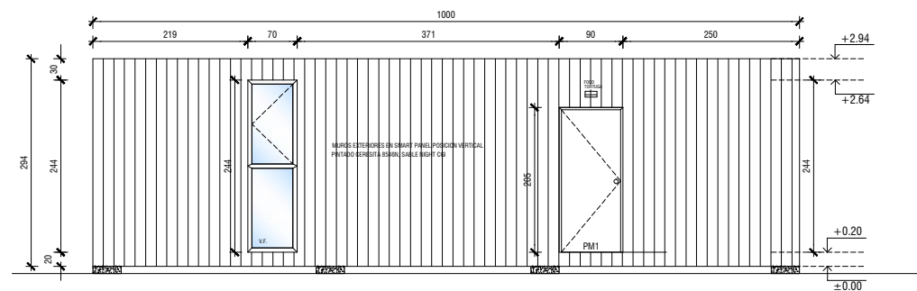
ELEVACION POSTERIOR
